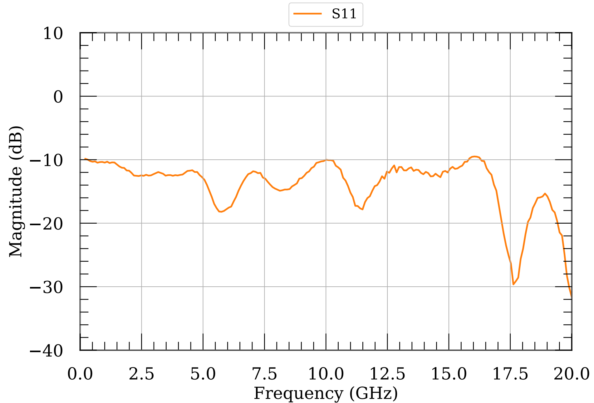
LNA S-params module088v2
